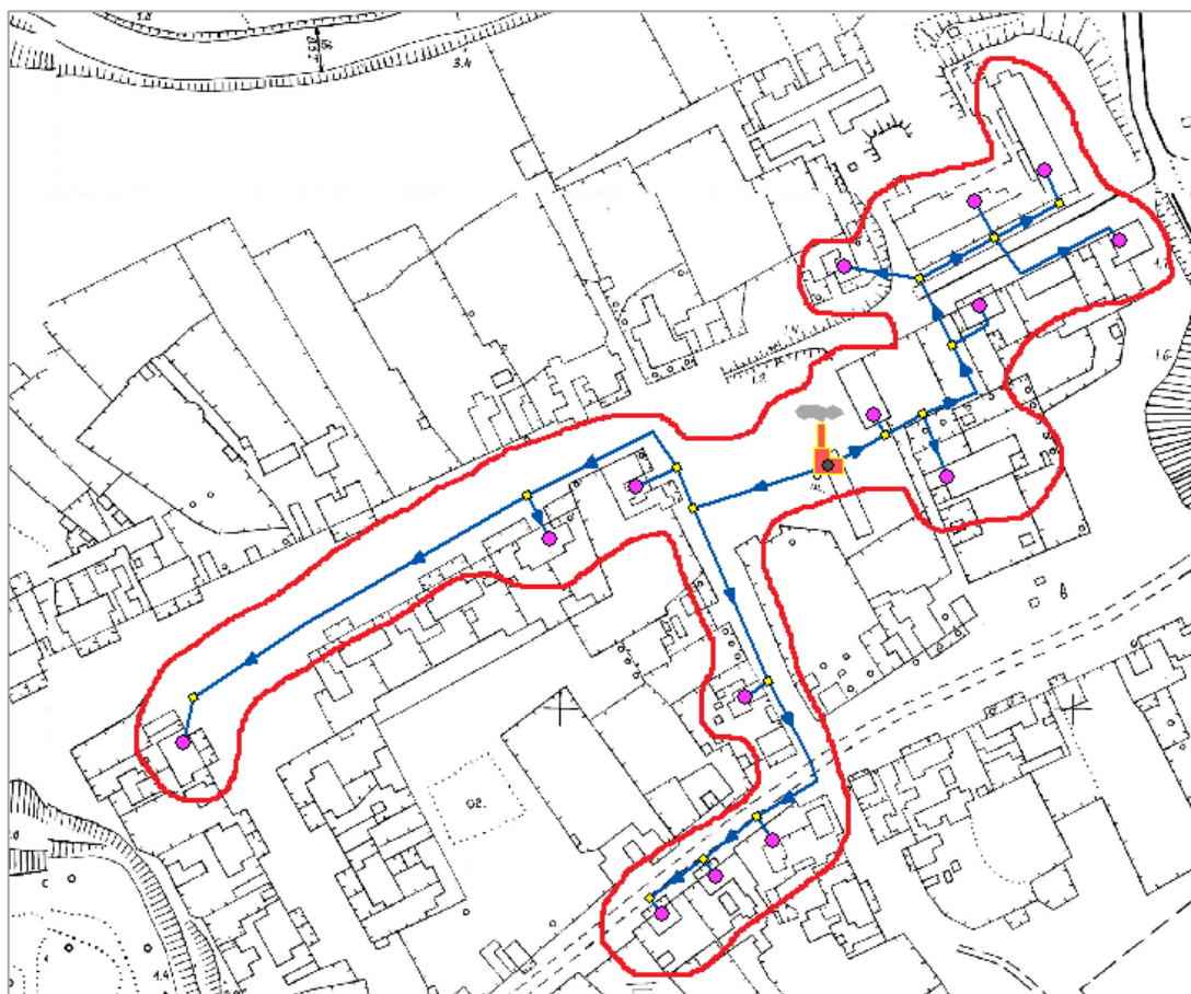
Рисунок 29. Зона действия котельной № 4, д. Шипицына
