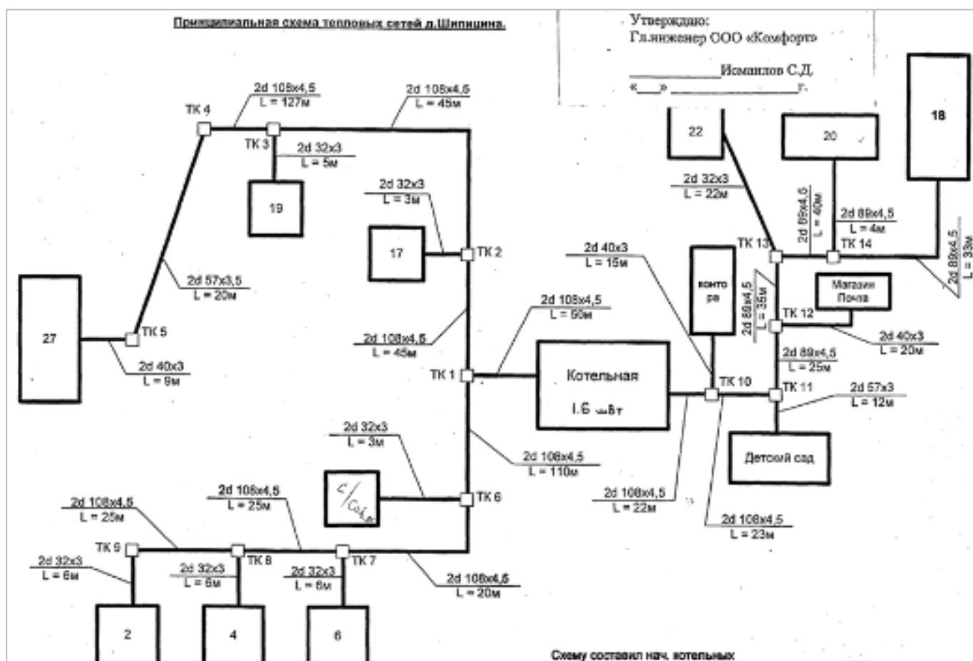
Рисунок 18. Бумажная схема тепловой сети от котельной № 4, д. Шипицына
