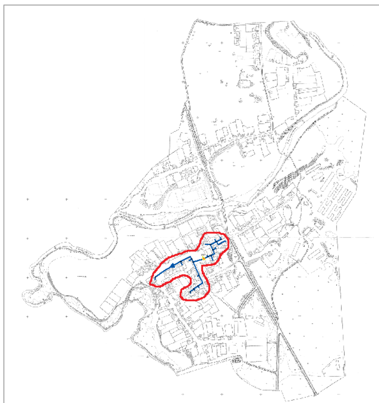
Рисунок 37. Зоны нормативной и ненормативной надежности и безопасности теплоснабжения д. Шипицына (красным цветом выделены зоны ненормативной надежности и безопасности теплоснабжения)
